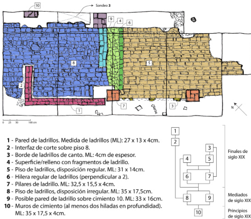
Figura 8 - Esquema en planta de las estructuras halladas en el Patio de Chacareros. Los colores indican distintas unidades estratigráficas, cuya relación y cronología se analizan en la matriz.
