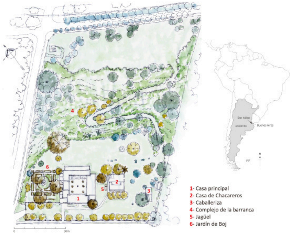
Figura 1. Planta esquemática del conjunto donde se indican las unidades principales (dibujo de Jorge Bayá Casal, Archivo Museo Pueyrredón). A la derecha, mapa de Sudamérica con la ubicación del sitio.
